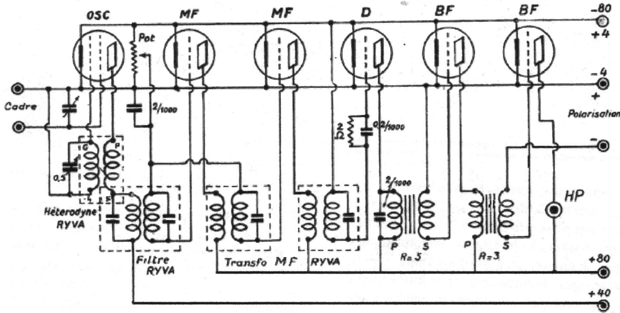
Selbstschwingender Mischer Modulateur Bigrille
